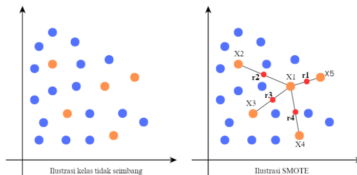
Gambar 2. Ilustrasi SMOTE
